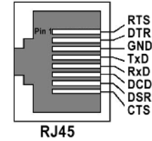
RJ45
