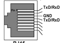
RJ45
